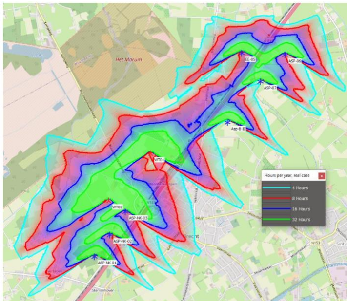
Figuur 1-4: Overzicht projectgebied met cumulatieve slagschaduw ISO contouren (uren per jaar verwachte slagschaduw, vergunde situatie + turbines Brecht Hoekakker)
